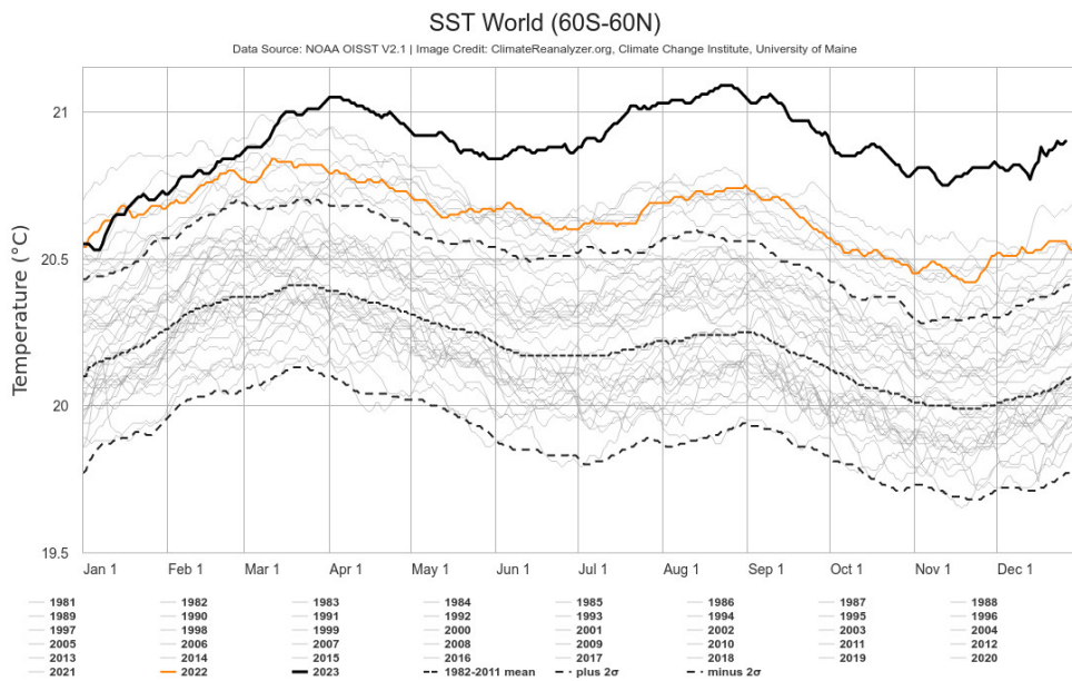
Figura 1: Temperatura del mar. Dades extretes de NOAA OISST V2.1 https://psl.noaa.gov/data/gridded/data.noaa.oisst.v2.html
